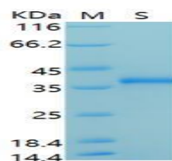
SDS-PAGE Result
