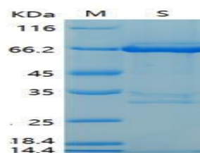
SDS-PAGE Result
