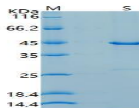
SDS-PAGE Result
